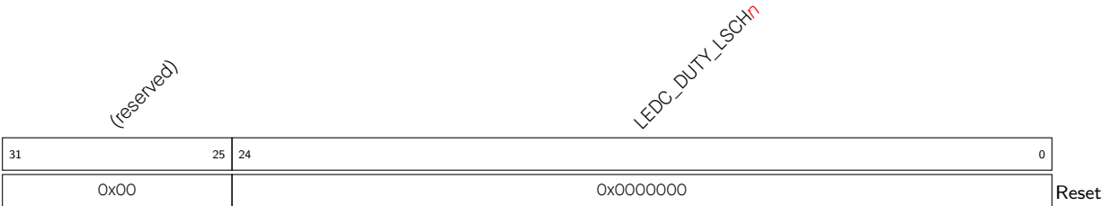
Register 28.8. LEDC_LSCH n _DUTY_REG ( n : 0-7) (0xA8+0x14* n )
